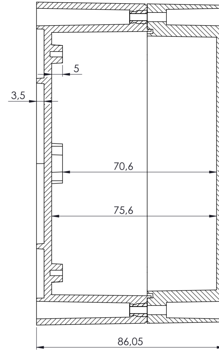
KESIT A-A
