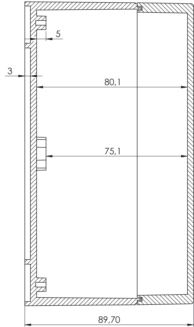
KESIT A-A
