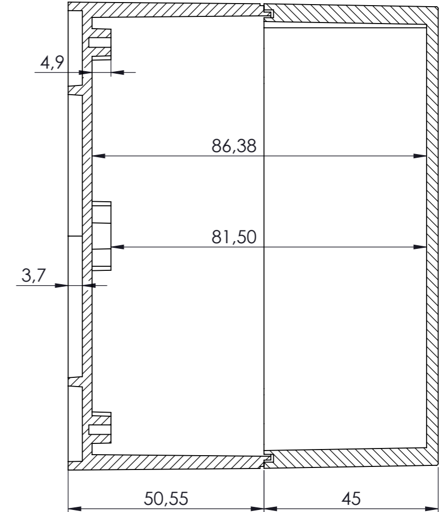
KESIT B-B
